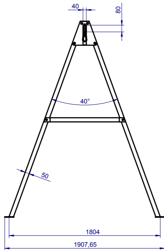
PRZEKRÓJ A-A
